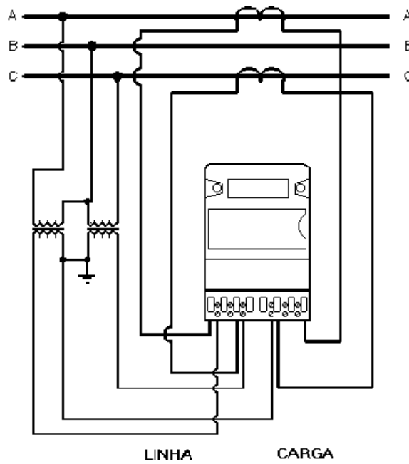
Figura 6.2 - Ligação Medição Indireta a 2 elementos com TC e TP
